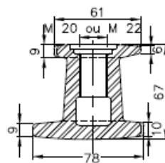
Coupe A-A
