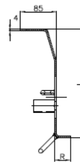
Coupe A-A
