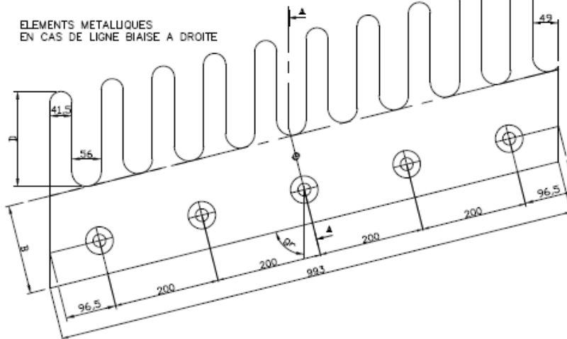
Châssis
